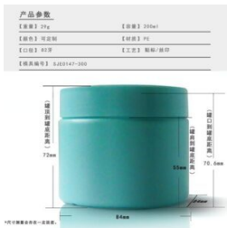
SJE0147-300 300ml PE Bottle Material: PE Capacity: 300
