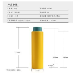
SJE1641-500 500ml PE Bottle Material: PE Capacity: 500
