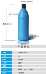
SJE0169-900 900ml PE Bottle Material: PE Capacity: 900
